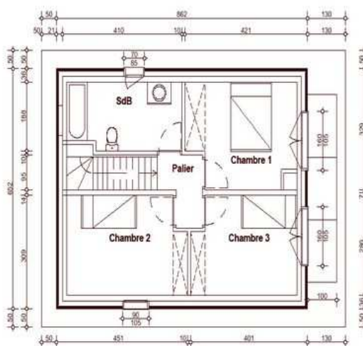
Étage 1/50
